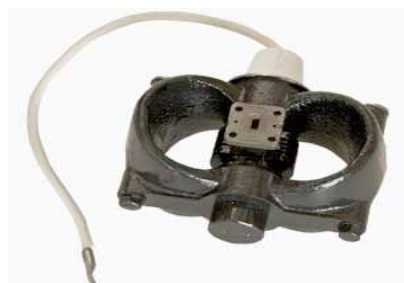
10 Пакетированный магнетрон, черные скобы — магниты ( сайт http://istok2.com )
